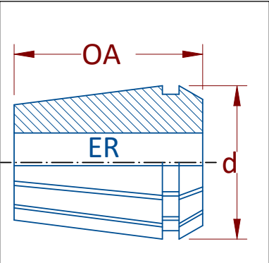
ER Collet
